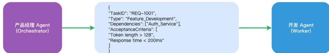
A2A 协议架构
