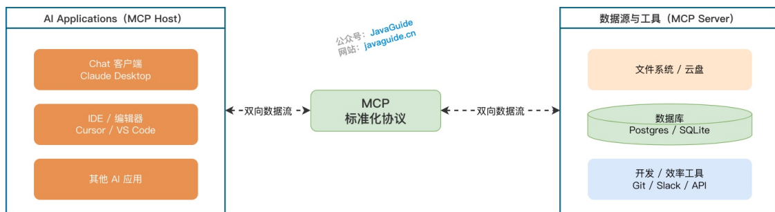
MCP 图解
